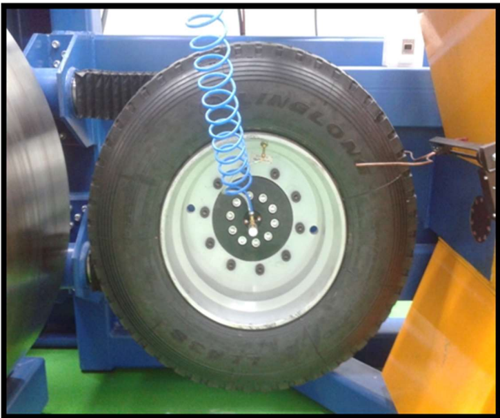
เครื่องทดสอบสมรรถนะความเร็วการรับโหลด รถบรรทุกและรถโดยสาร (มอก.2719, UN R 54)
